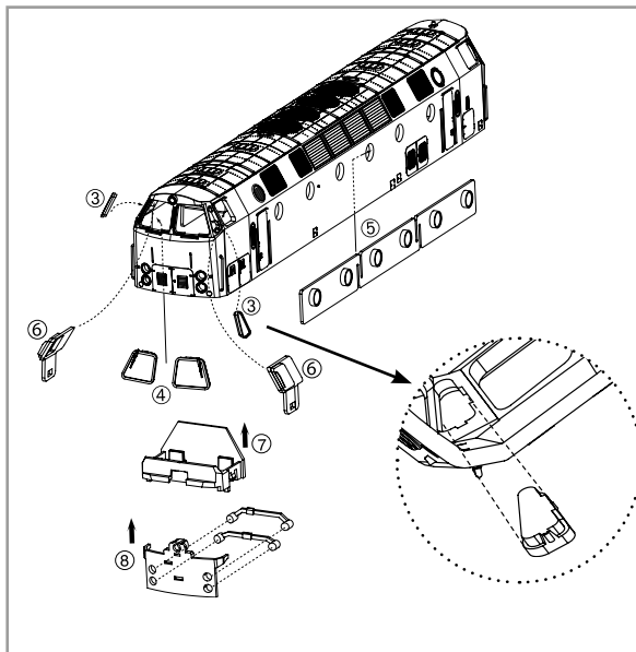
Führerstand-Demontage Drivers cab-disassembly Cabine de conduite-démontage
